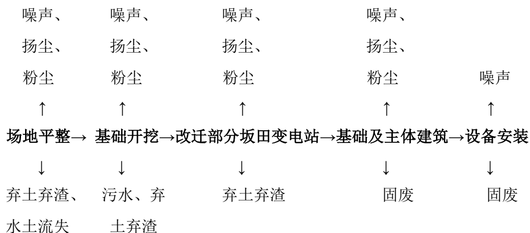
图 1 施工期工艺流程图
